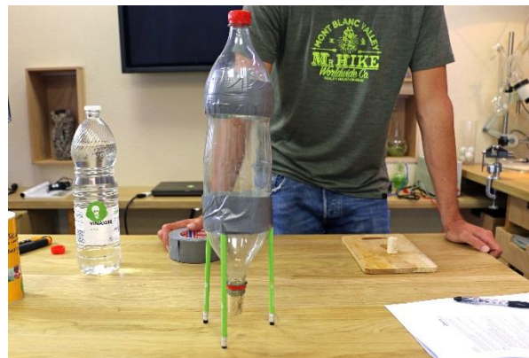
d. Die Rakete ist nun fertig.
