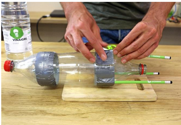
c. Klebe die Bleistifte in ungefähr gleichem Abstand am Boden der ganzen PET-Flasche fest, so dass die Flasche und die Bleistifte etwa 15 cm überlappen. Die Spitze der Bleistifte sollte zu der Spitze der Rakete zeigen.
